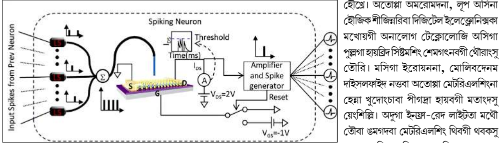
ন্যুরোমোর্ফিক চিপকী সার্কিট দাইএগ্রাম
